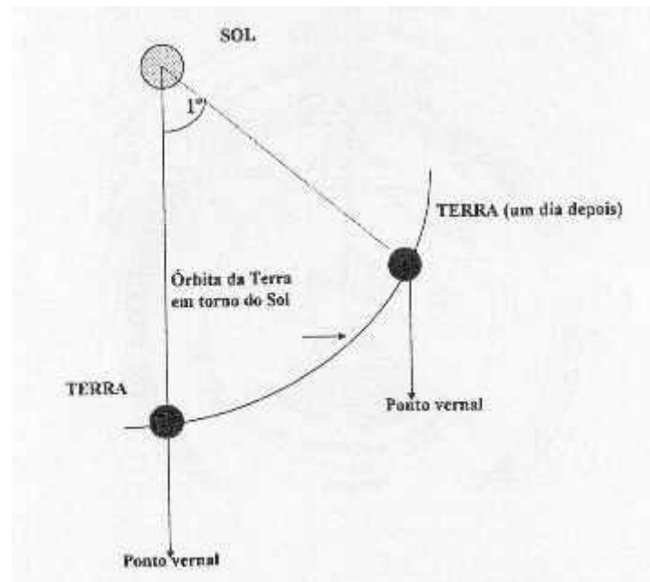
FIGURA 3: A Terra, no seu movimento em torno do Sol, desloca-se 1^\circ por dia, o que provoca uma ligeira diferença entre o Dia Solar e o Dia Sideral.
