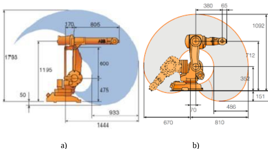
Figura 8: Volume de trabalho de um robô [22].
