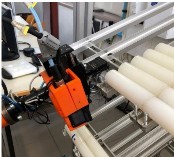
Figura 64: Ausência de peça na coluna dois do armazém.
