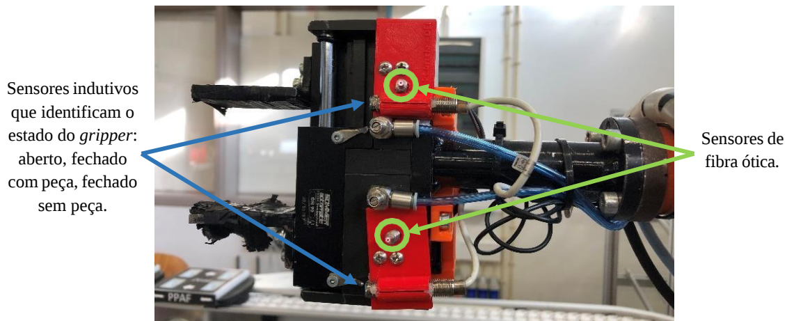
Figura 16: Gripper do robô IRB 1400.
