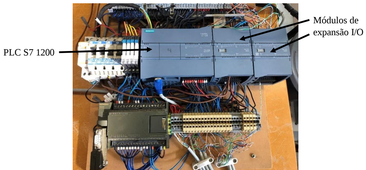
Figura 36: Gestor da CFF - PLC S7 1200.
