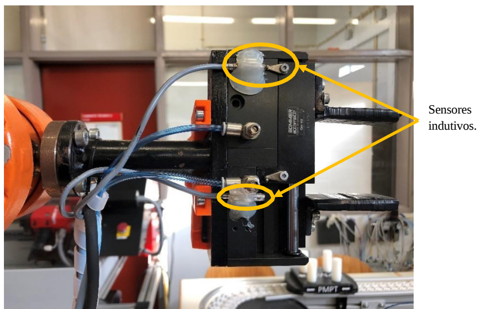
Figura 19: Ferramenta de trabalho IRB 140.
