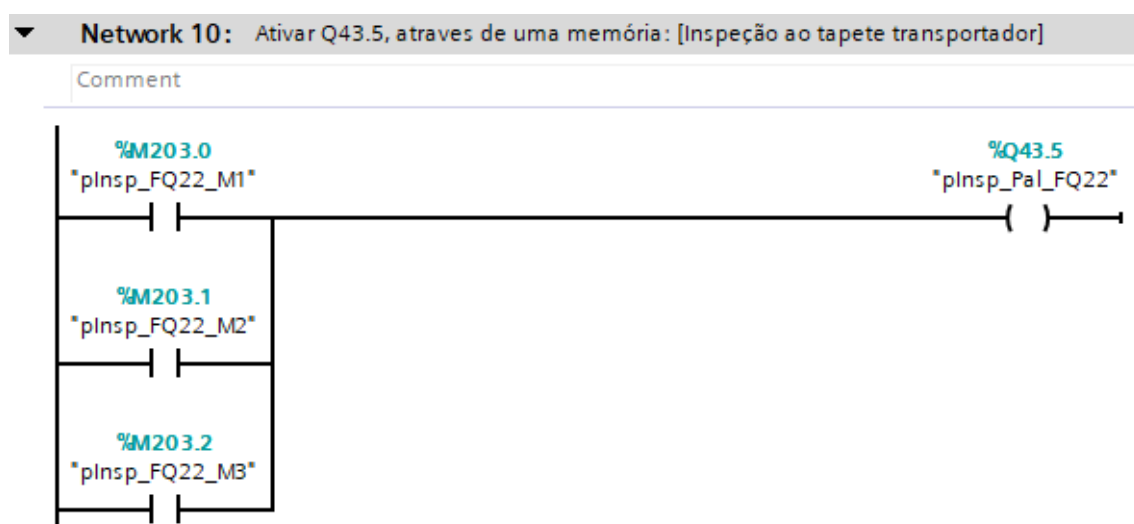
Figura 96: Ativação da saída Q43.5 do autómato.
