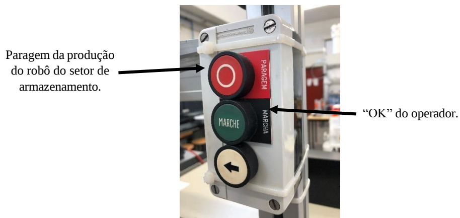
Figura 30: Botoneira do setor de armazenamento.
