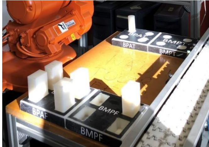
Figura 20: Buffer de peças do setor de fabrico.
