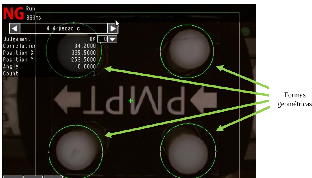
Figura 97: Definição das formas geométricas no software TouchFinder .
