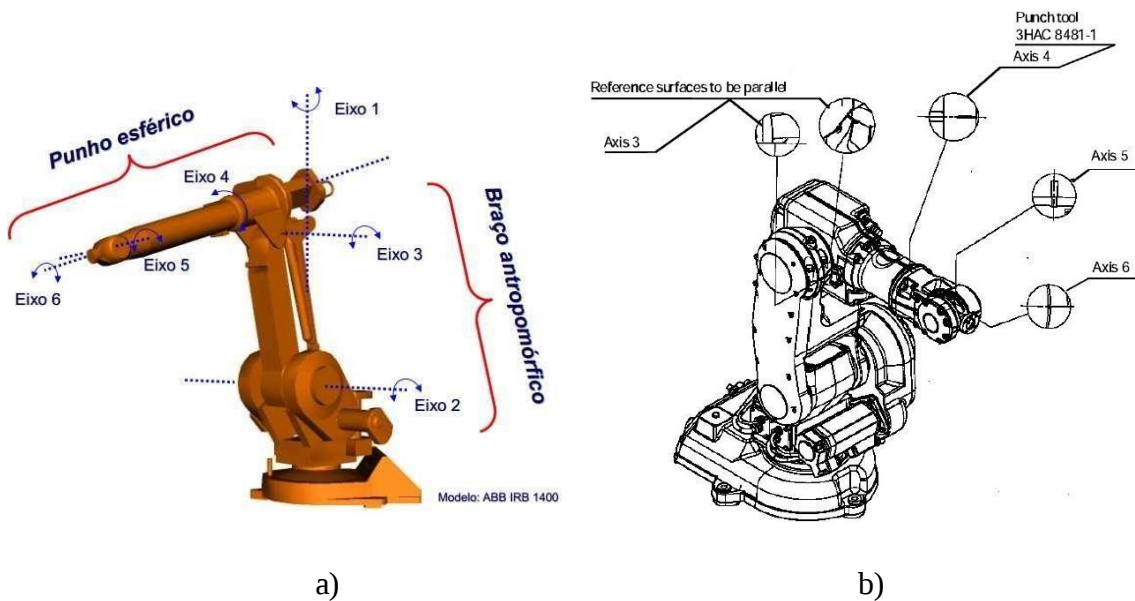
Figura 9: Juntas de um robô.
