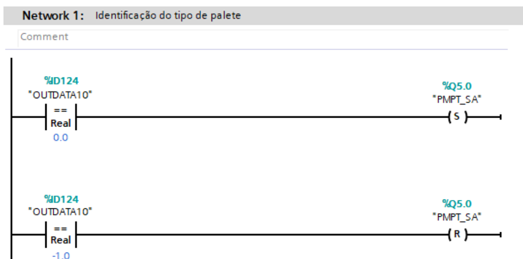
Figura 89: Tratamento de dados e identificação do tipo de paleta.
