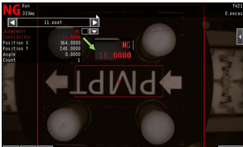
Figura 85: Identificação da sigla PMPT com correlação NOK.
