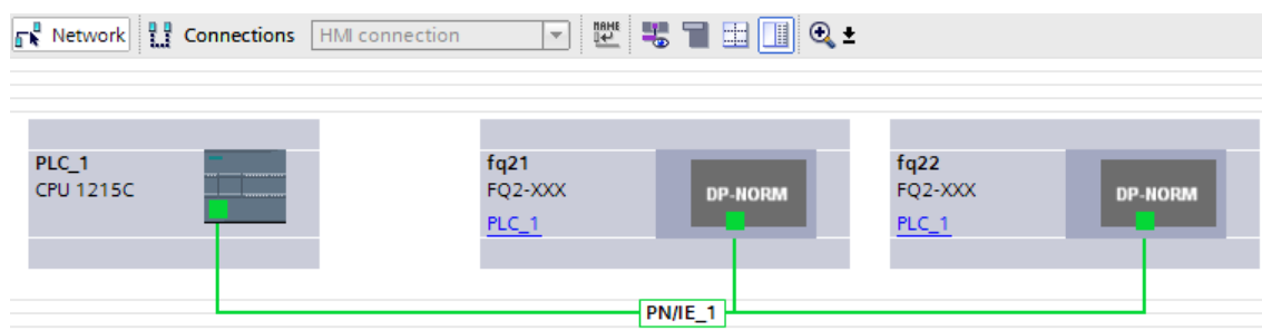
Figura 81: Comunicação entre PLC e Câmaras no TIA Portal.
