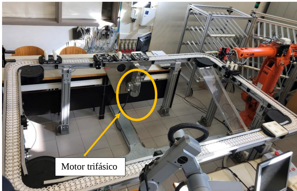
Figura 26: Sistema transportador da CFF.
