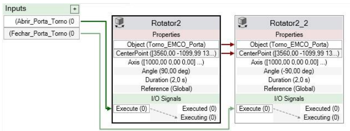
Figura 56: Simulação de abertura e fecho da porta do torno.
