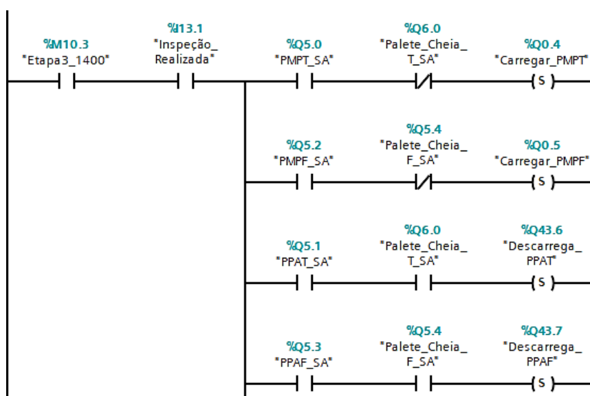
Figura 40: Código de programação no TIA Portal.
