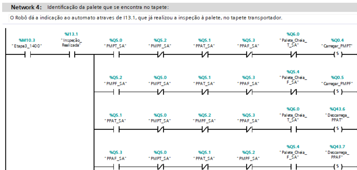
Figura 92: Identificação da paleta no SA.
