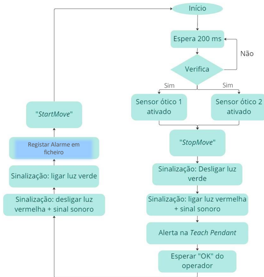
Figura 32: Diagrama de blocos da multitask .
