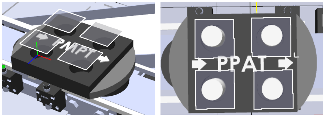
Figura 51: Plane Sensors instalados nas paletes.
