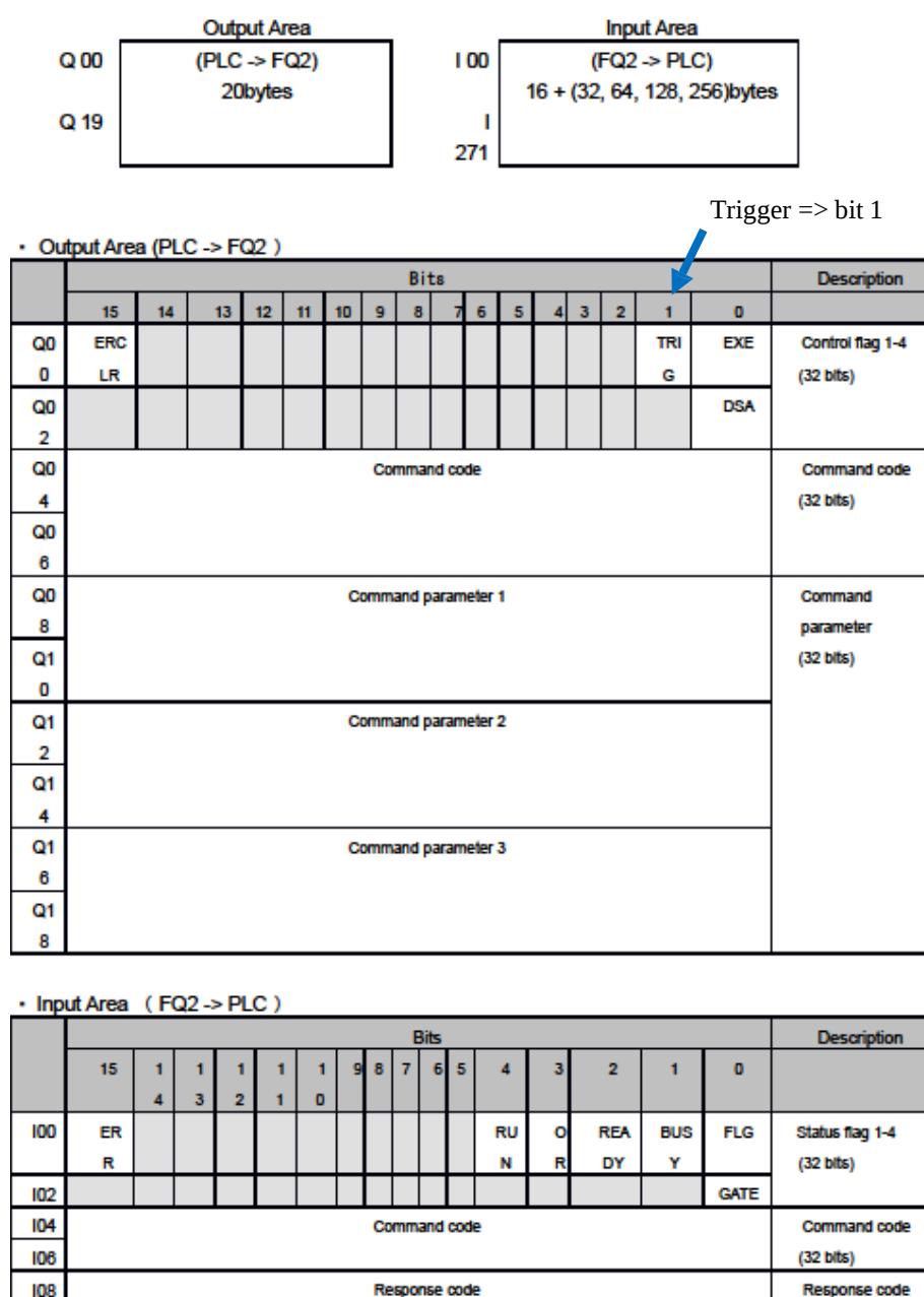
Figura B-1: Endereços de memória do sistema de visão FQ2.
