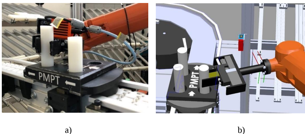
Figura 63: Carregamento da PMPT.
