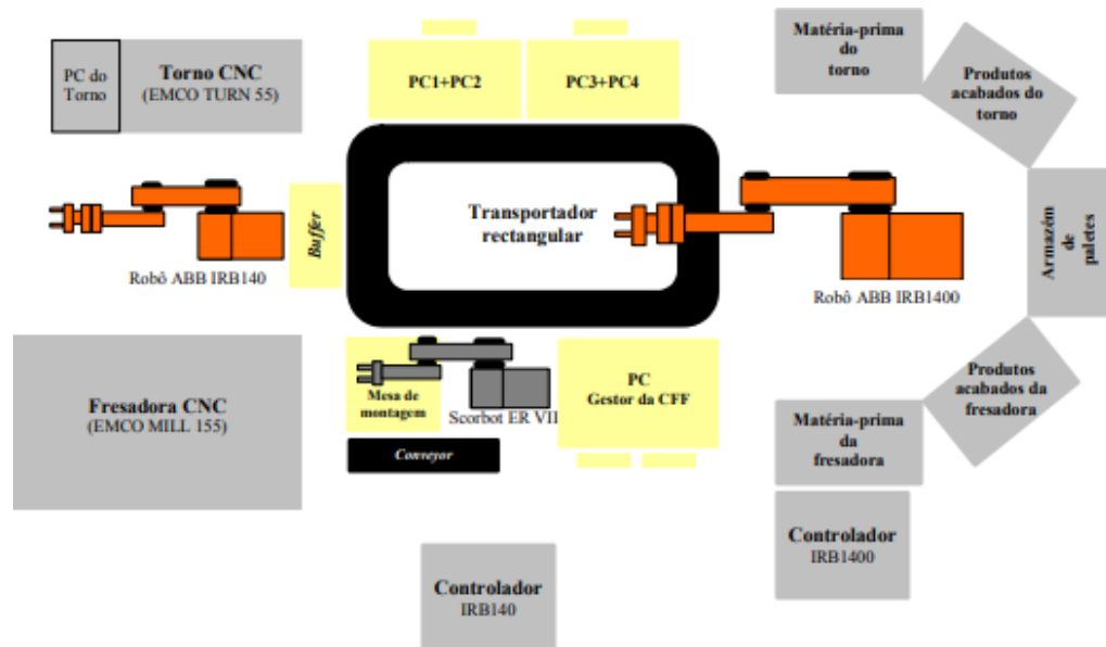
Figura 12: Layout da CFF do laboratório [15].
