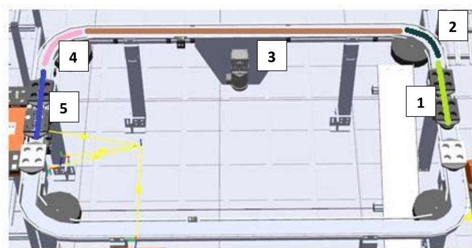
Figura 53: Sistema transportador.
