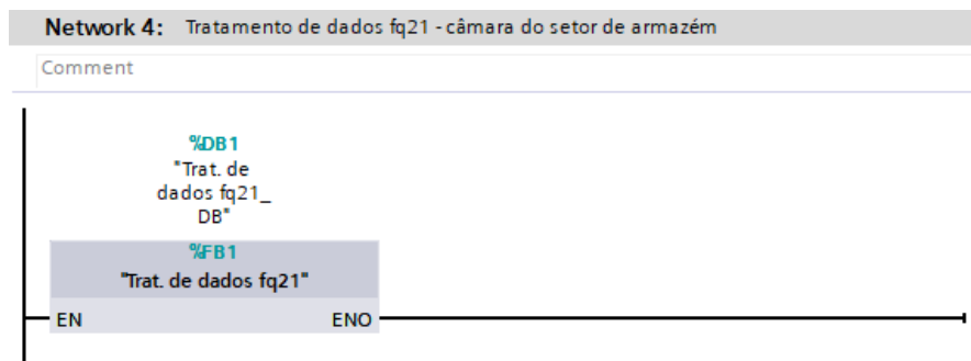
Figura 88: Function Block do tratamento de dados da câmara fq21.
