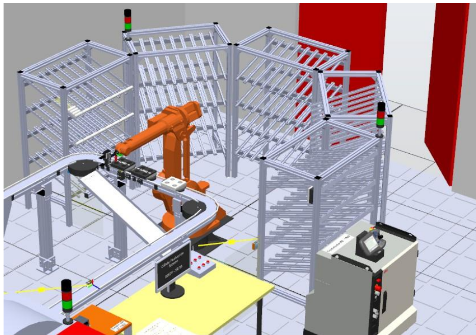
Figura 46: Representação do setor de armazém no RobotStudio .
