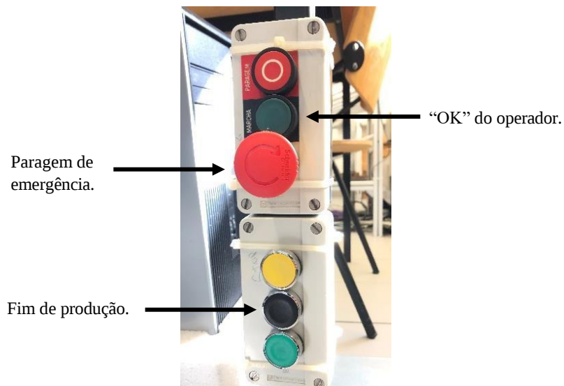
Figura 29: Botoneira do setor de fabrico.
