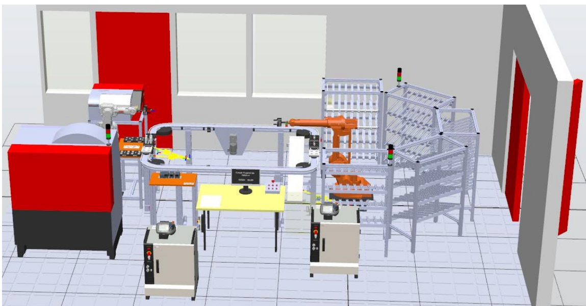
Figura 47: Visão geral da CFF no RobotStudio .
