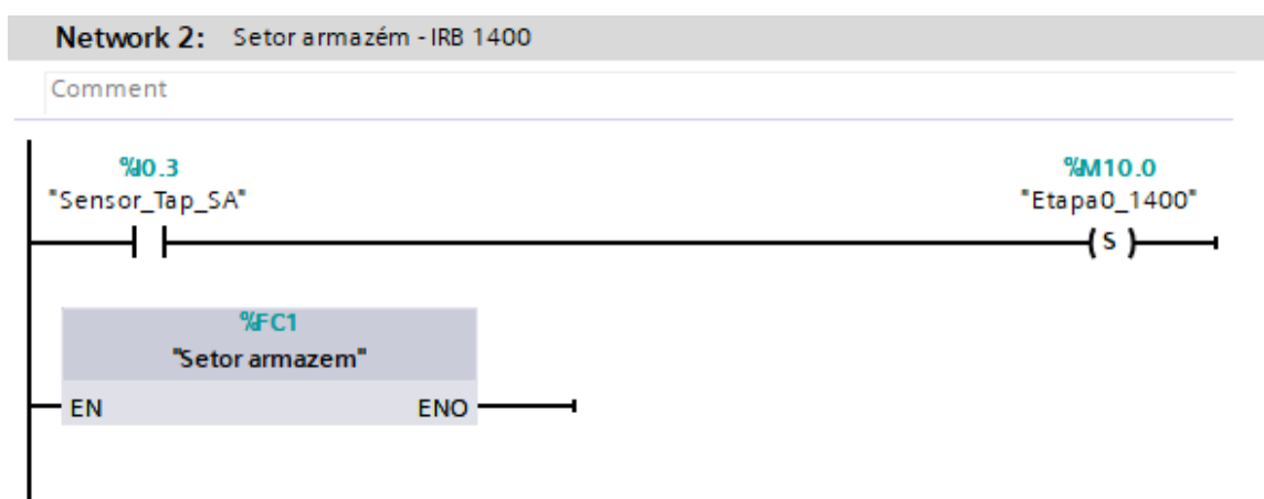
Figura 94: Network do setor armazém.
