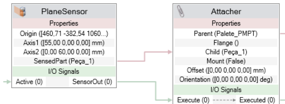
Figura 52: Desenvolvimento de Smart Components .
