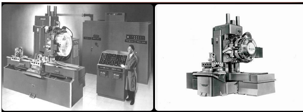
Figura 11: Primeira fresadora NC [25].
