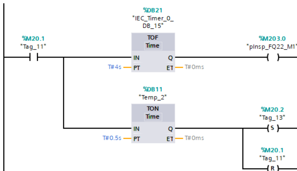
Figura 95: Network responsável pela inspeção à paleta no SA.
