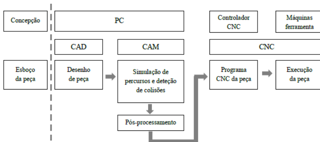
Figura 23: Funcionamento CAD/CAM/CNC [15].
