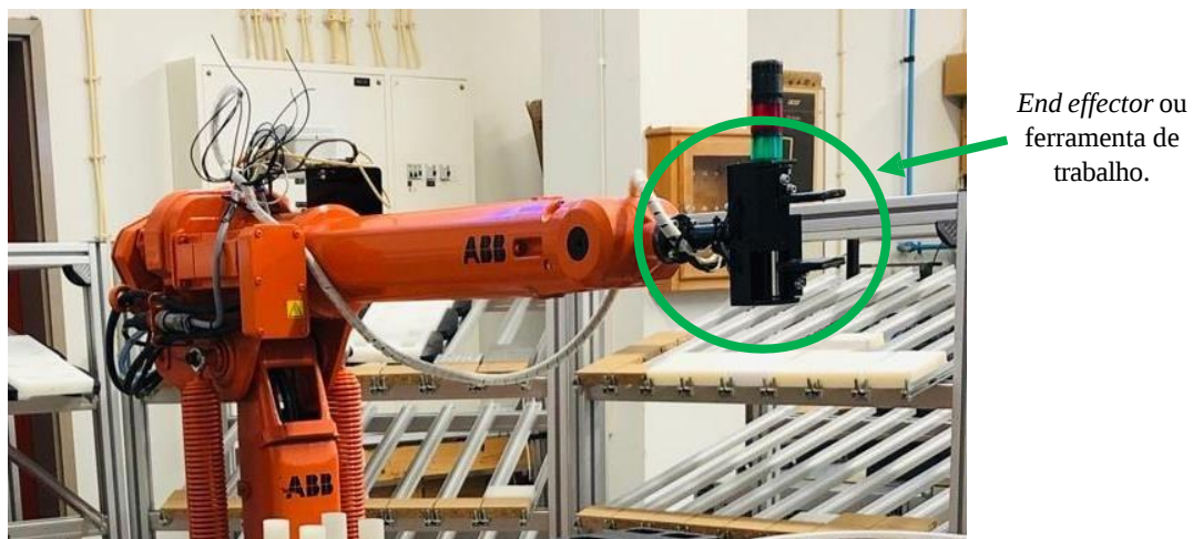
Figura 6: End effector do robô IRB 1400 do Laboratório de Automação e Robótica [19].
