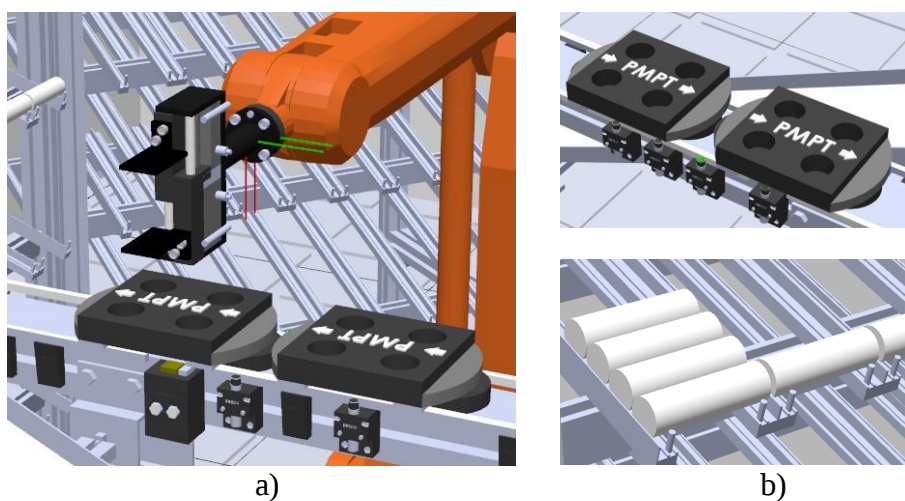
Figura 43: Elementos desenvolvidos no software de desenho.
