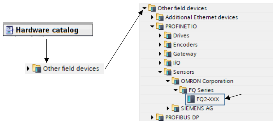
Figura 82: Adicionar a biblioteca da câmara FQ2 no TIA Portal.
